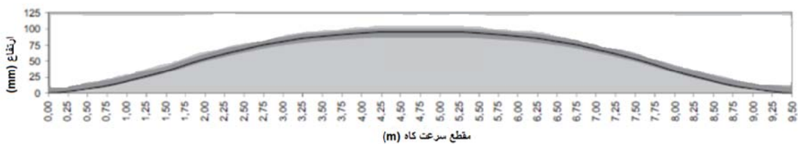
شکل ۳-۴۸-ب-مقطع عرضی سرعت‌گاه سینوسی با سرعت ۵۰ کیلومتر در ساعت
