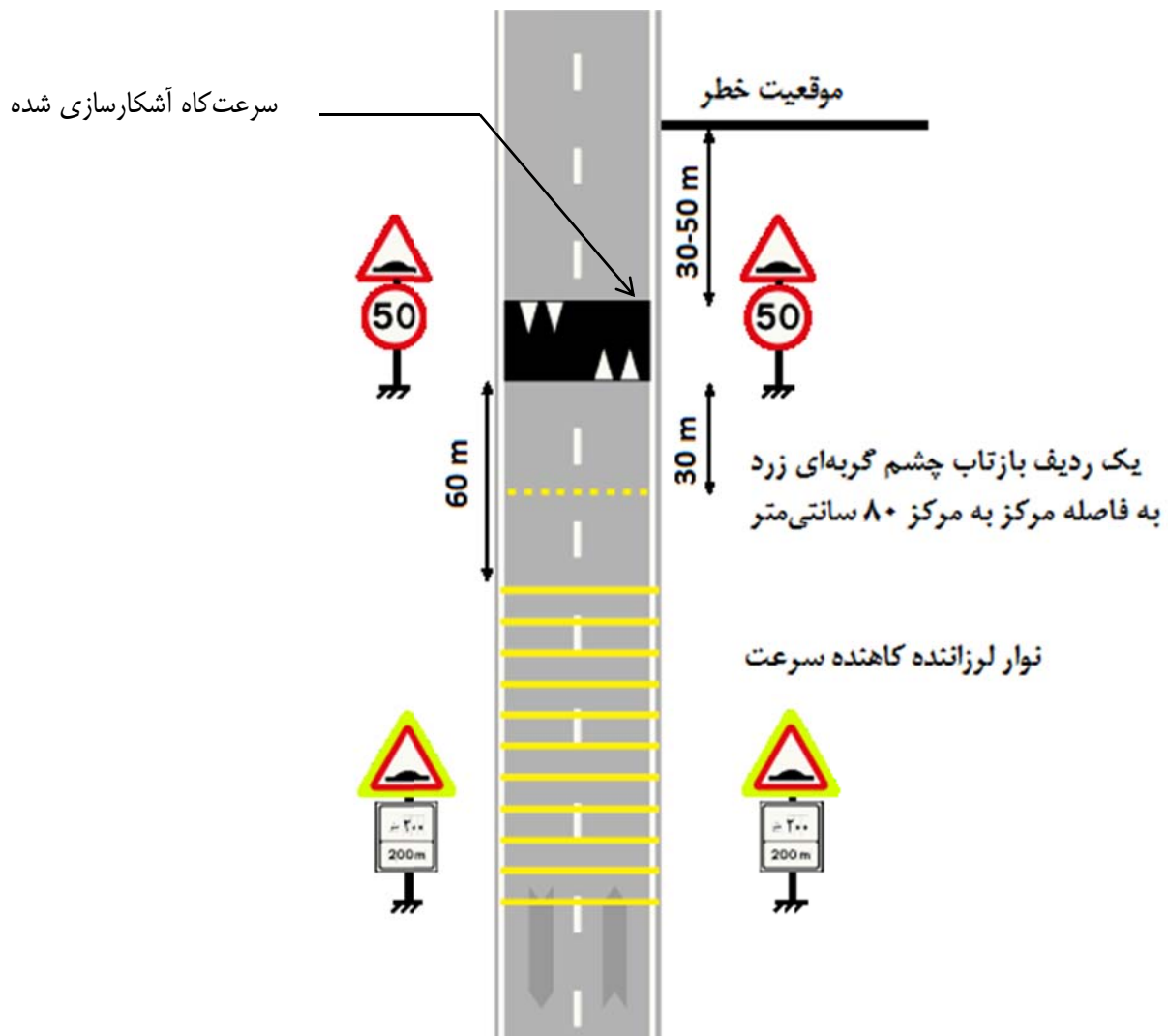
شکل ۳-۴۸-الف-نمونه‌ای از طرح سرعت‌گاه در راه‌ها، ده‌خطه
