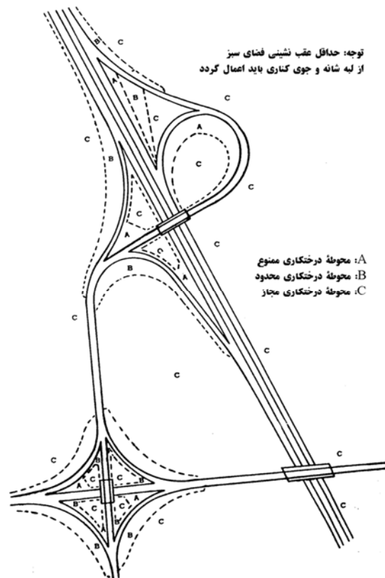
شکل ۳-۴۵- محدوددهای مجاز و ممنوع درختکاری در محوطه یک تبادل
