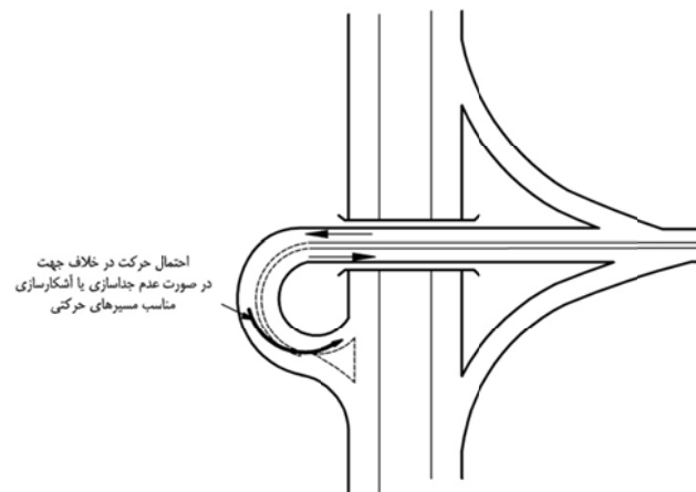
شکل ۳-۳۷- احتمال حرکت اشتباه در صورت عدم جداسازی مسیره‌های حرکت در داخل گردراهه
